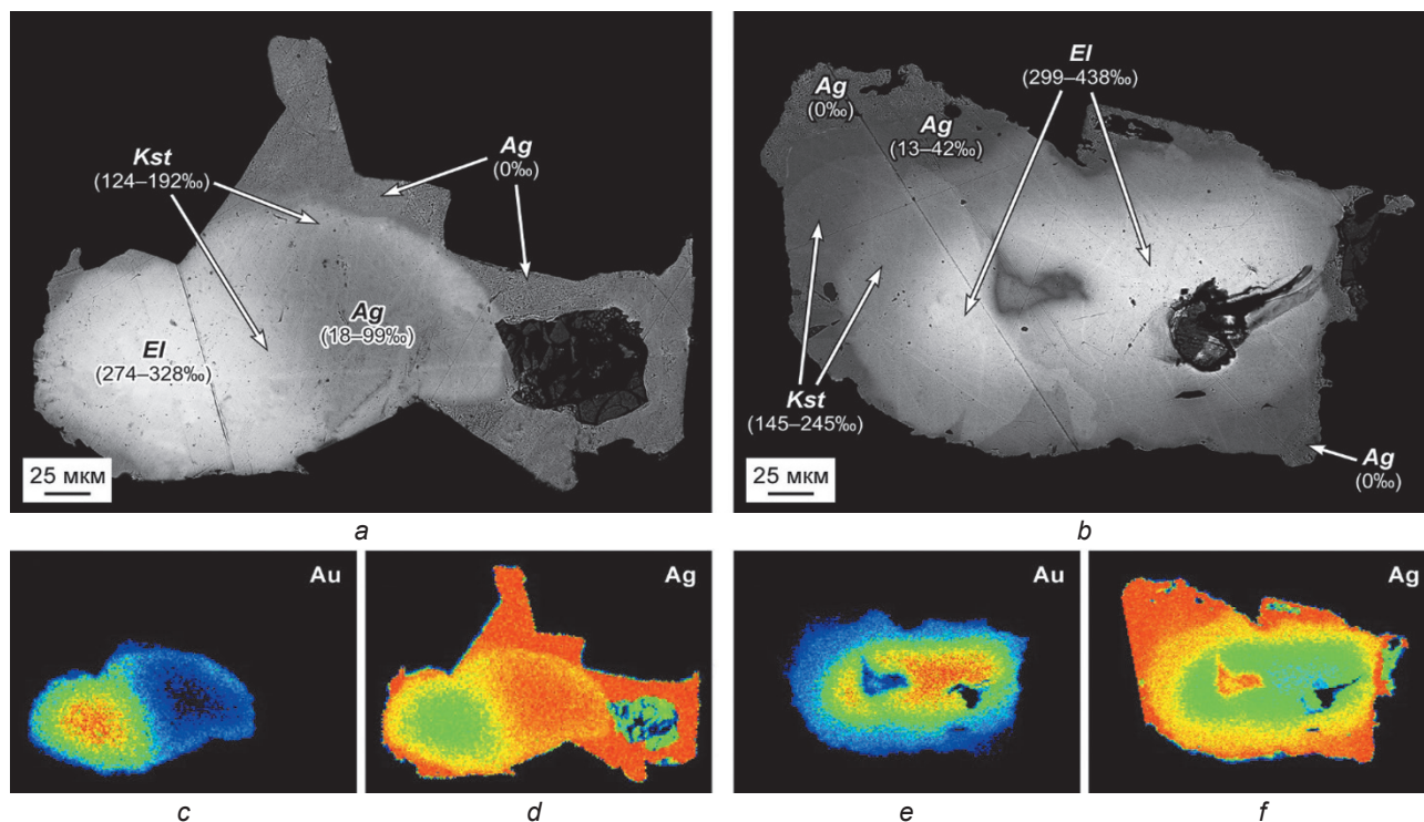
Рис. 2. Неоднородность основного состава золото-серебряных частиц: изображения даны в обратно рассеянных электронах (а, б),
