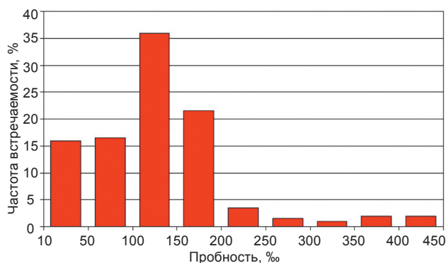
Рис. 1. Гистограмма пробности золото-серебряных частиц из руд преимущественно серебряного состава, месторождение Дука́т (количество замеров – 200) Fig. 1. Fineness histogram of gold-silver particles from ores of predominantly silver composition, Dukat deposit (number of measurements – 200)
