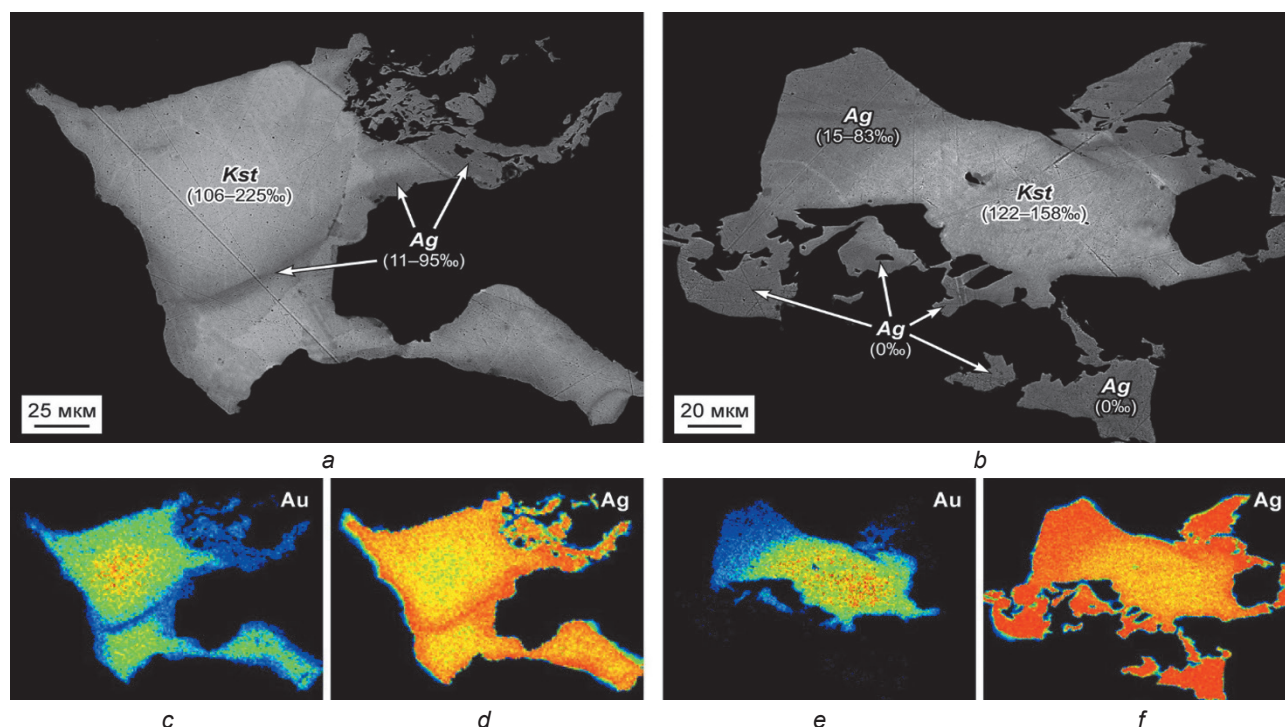
Рис. 5. Зональные зерна, состоящие из кустелита и самородного серебра: изображения даны в обратно рассеянных электронах (а, б), в рентгеновских лучах золота (с, е) и в рентгеновских лучах серебра (д, ф)
