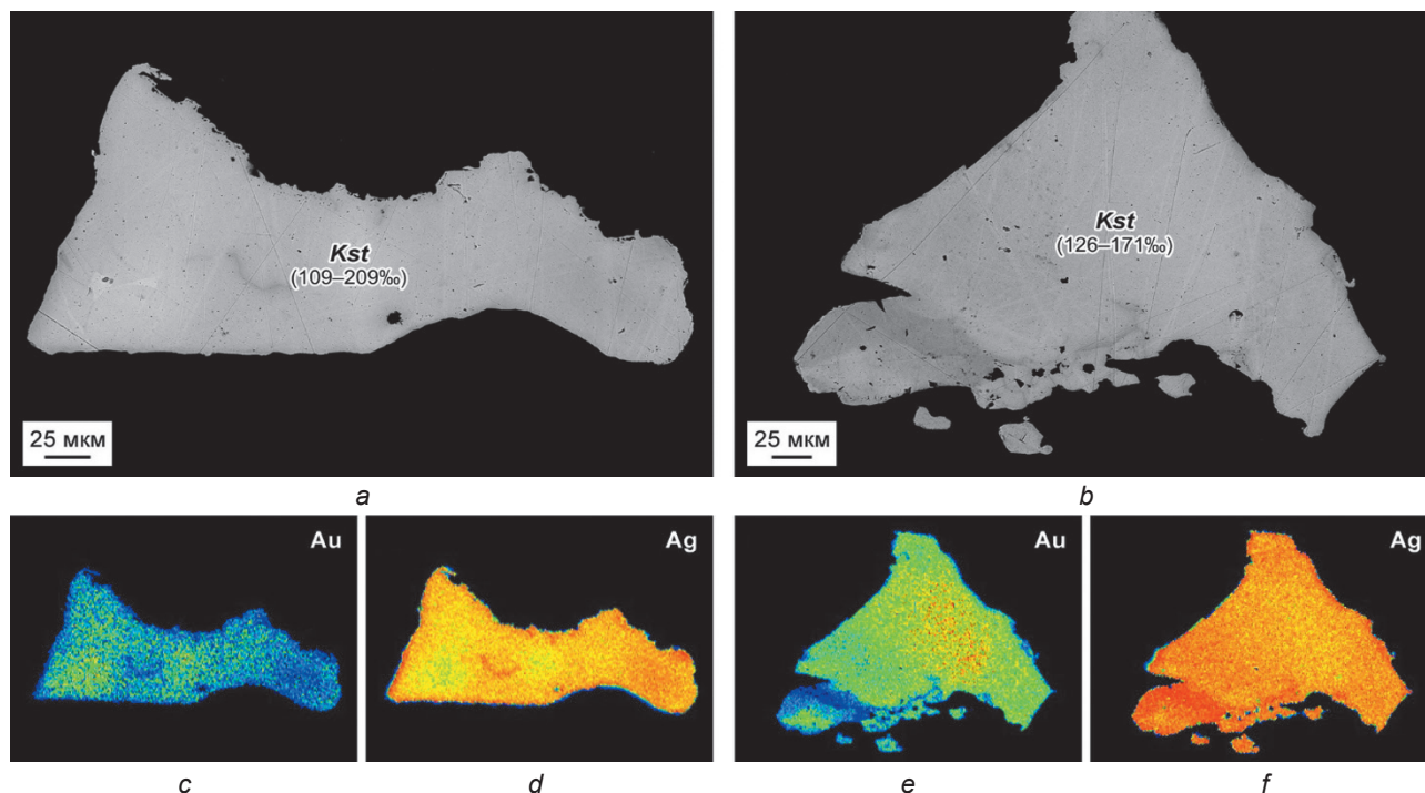
Рис. 3. Зерна кюстелита:
