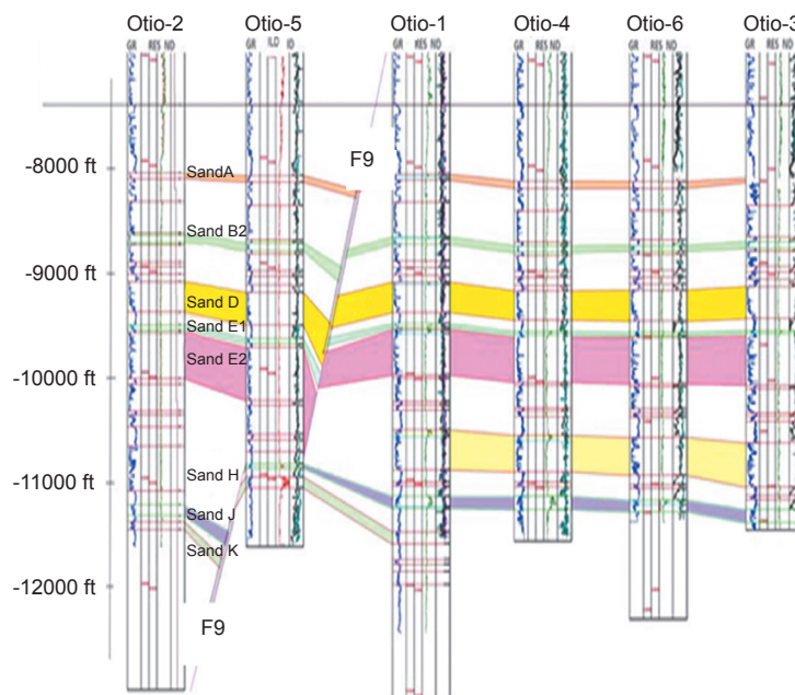
Fig. 17. Sand to sand correlation of the "Otio Field" (Powerlog, 2014) Рис. 17. Взаимосвязь между песками месторождения Отио (Powerlog, 2014)
