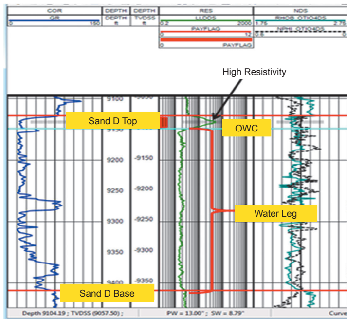
Fig. 13. Sands D in Otio-1 with high resistivity interpreted as hydrocarbon zone (Powerlog, 2014) Рис. 13. Пески D в Отио-1 с высоким каротажем сопротивления, рассматриваемые как углеводородная зона (Powerlog, 2014)
