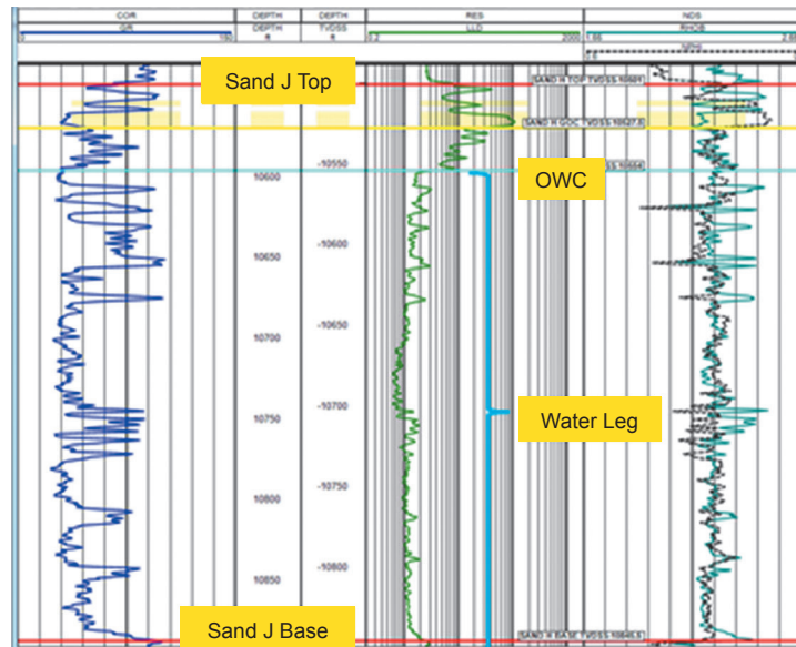
Fig. 16. Sands J in Otio-4 with high resistivity interpreted as hydrocarbon zones (Powerlog, 2014) Рис. 16. Пески J в Отио-4 с высоким каротажем сопротивления, рассматриваемые как углеводородные зоны (Powerlog, 2014)
